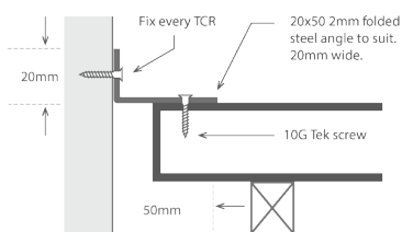
Detail A: TCR fixed edge
